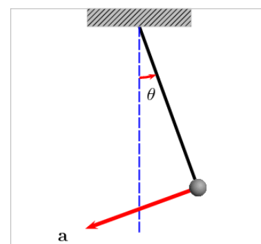
Obrázek 9: Obyčejné fyzikální kyvadlo
